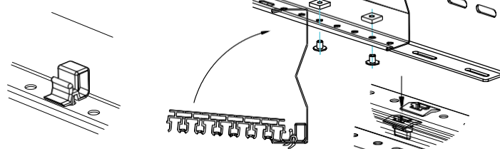
Защелка PR7-MCB в нижней части опорного профиля SP7
