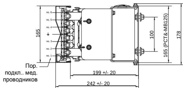
Опорный кронштейн РСТ7-MB125 для токоъемной тележки
